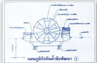
แผนภูมิกังหันน้ำชัยพัฒนา 1
